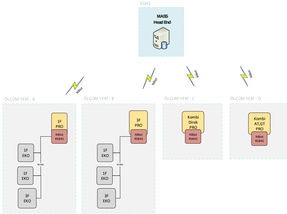
Figür 2 – NB-IoT tabanlı Pilot Proje Prensi Şeması
